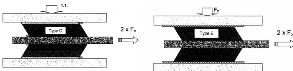
Σχ.3.3.5-2: Εργαστηριακή διάταξη προσδιορισμού μέτρου διάτμησης
