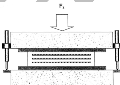
Σχ.3.3.5-1: Εργαστηριακή διάταξη προσδιορισμού μέτρου συμπίεσης
