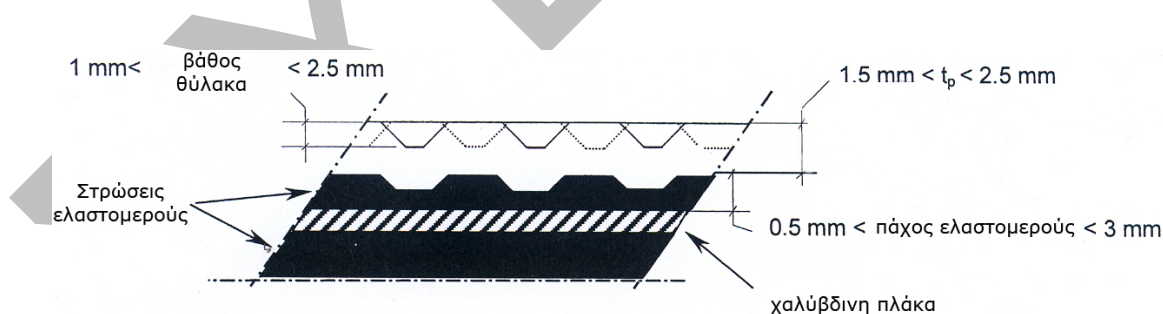
Σχ. 3.3.3-1: Τομή στην πάνω επιφάνεια ολίσθησης εφεδράνου τύπου D
