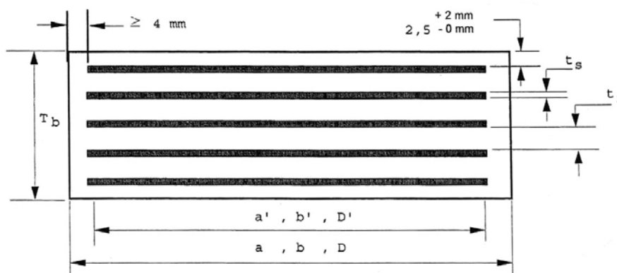
Σχ.2.1.1-1: Τυπική διατομή τυποποιημένου εφεδράνου τύπου Β
