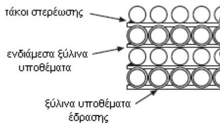
Διάταξη στοιβασίας σωλήνων (τομή)
