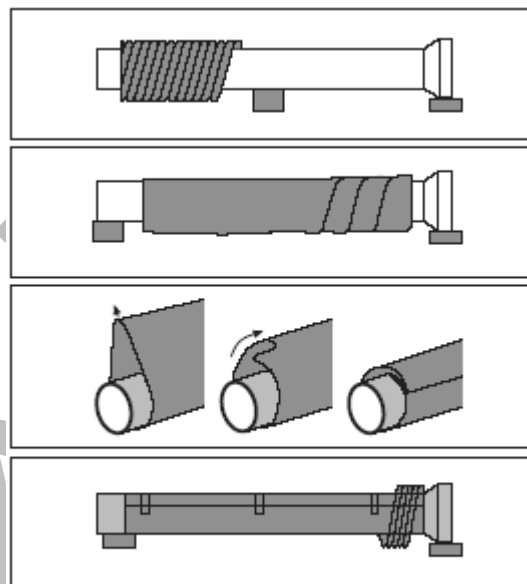
Διαδικασία εφαρμογής μανδύα πολυαιθυλενίου
