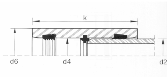
Σύνδεσμος τύπου REKA
