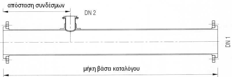
Αμφιφλαντζωτό στοιχείο με σύνδεση συναρμογής
