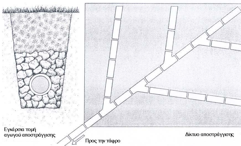
Εικ. 3-1. Αποστραγγιστικό δίκτυο. Εγκάρσια τομή όπου διακρίνεται η στρώση από γαρμπίλι, η τομή του σωλήνα και τα υλικά (σκύρα, γαρμπίλι) πλήρωσης των τάφρων. Κάτοψη του δικτύου με τους πλευρικούς αγωγούς να σχηματίζουν γωνία με τον κεντρικό (μορφή ψαροκόκαλου).
