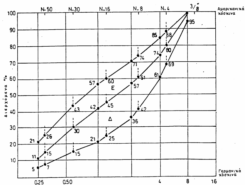
Διάγραμμα I : Ορια κοκκομετρικής διαβαθμίσης μίγματος αδρανών μεγίστου κόκκου □ 8 ή 3/8"
