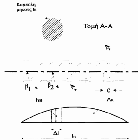
Σχήμα 3-4 Προσδιορισμός της ανηγμένης επιφάνειας προβολής, \alpha_R , των νευρώσεων
